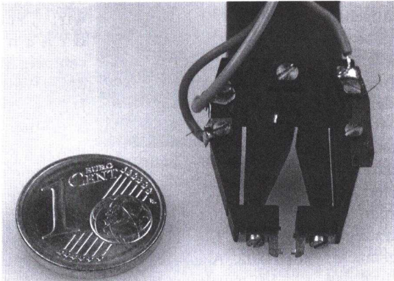
Entwicklung von Mikrogreifern für die Montage von Kleinstbauteilenm.
